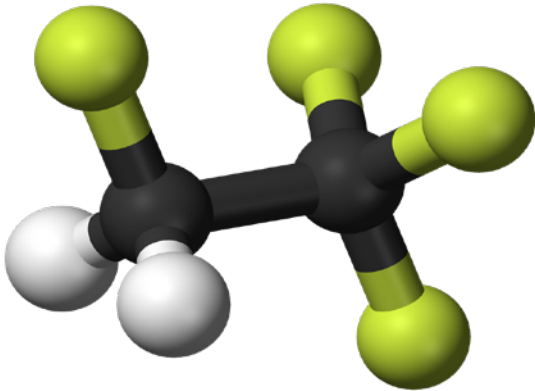
HFC R134a. Svart kol, gult väte och vit fluor.
