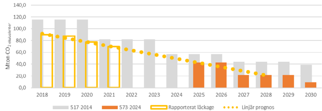
Utfasning av HFC köldmedier som får säljas inom EU. Orange visar den nya förordningen och grått den tidigare.
